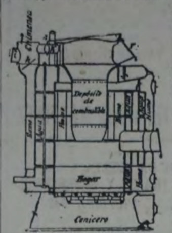
Fig. 1. Caldera Mamelle construida de hierro, para la calefacción por vapor a baja presión.
