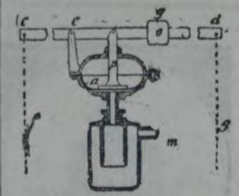
Fig. 2. Regulador de combustión para calderas a emplearse en la calefacción por vapor a baja presión.
